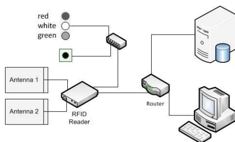
Fig. 2 RFID portal
